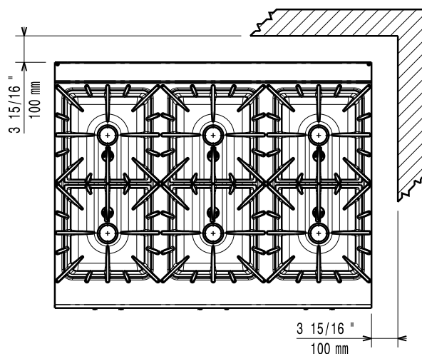
Päältä
