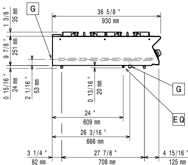
Sivulta
